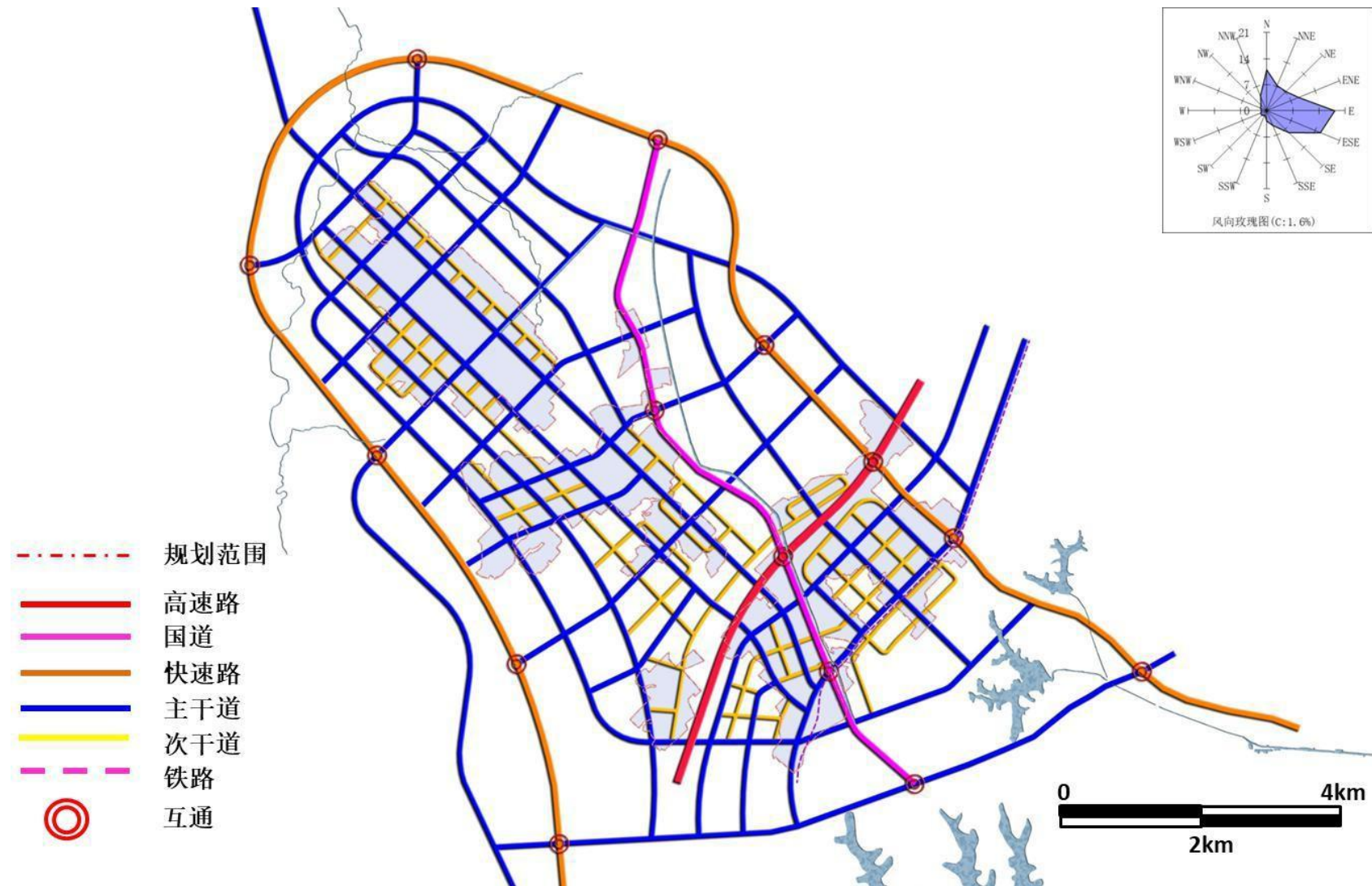
图 2.1-6 道路规划图
