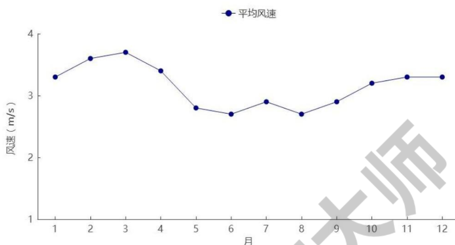
图 5.4-4 平均风速月际变化
