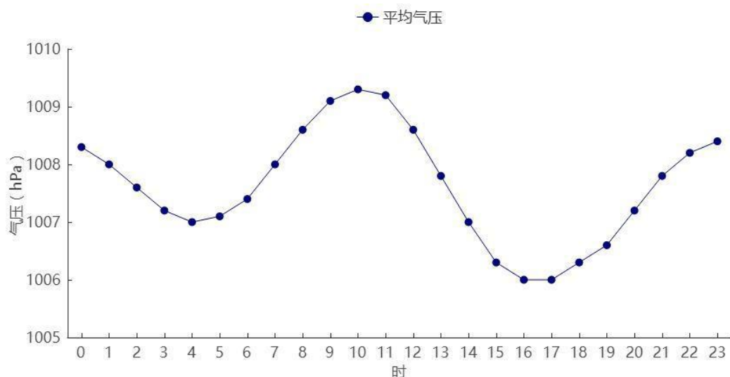
图 6.3-6 平均气压日变化
