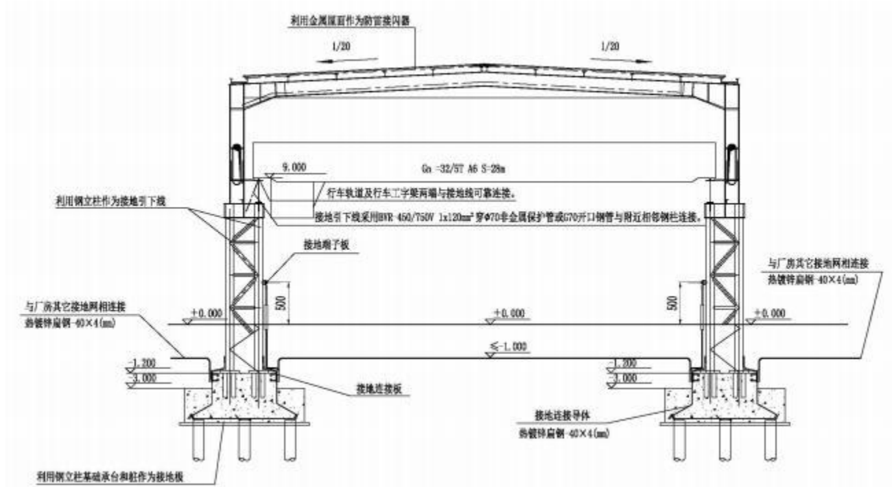
图8.2-1 钢结构厂房防雷示意图
