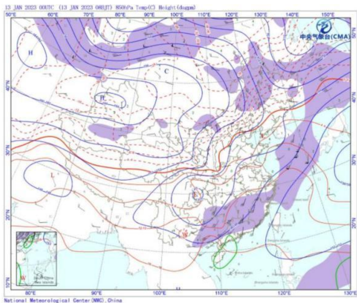
图6.1-6850百帕切变线
