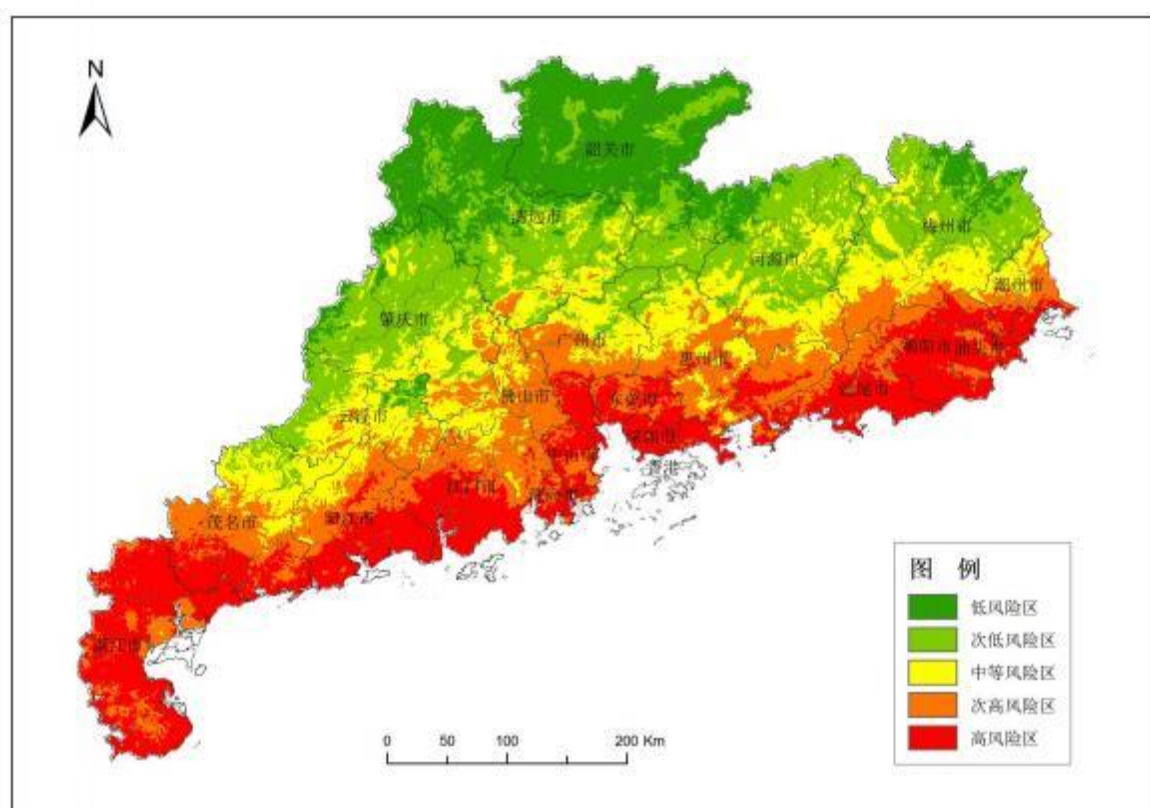
图4-1雷电风险区
