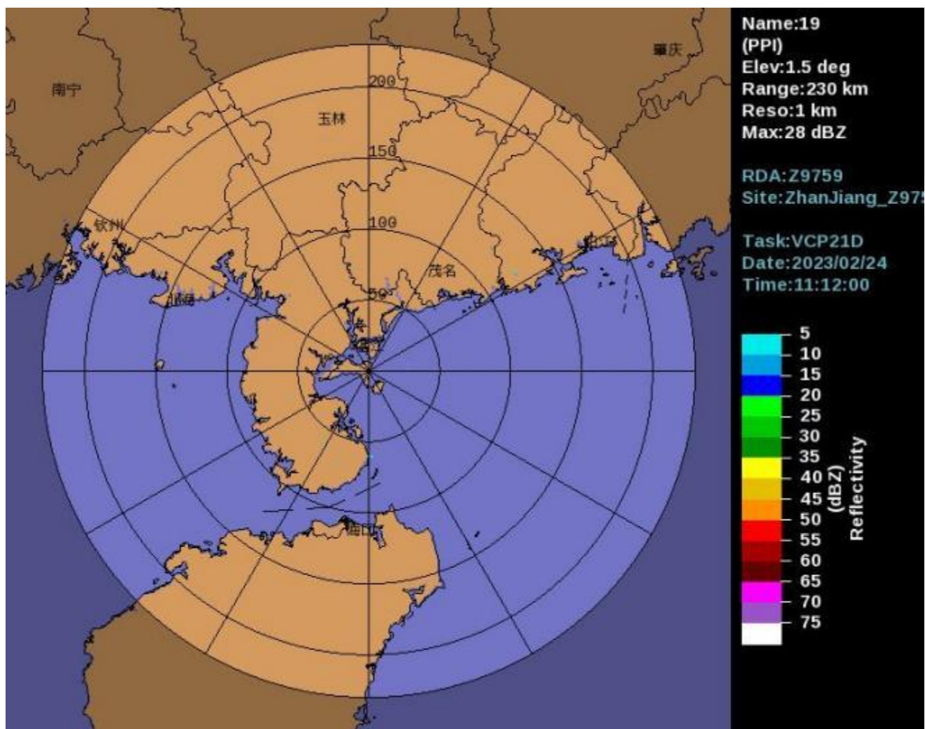
图6.1-2雷达图
